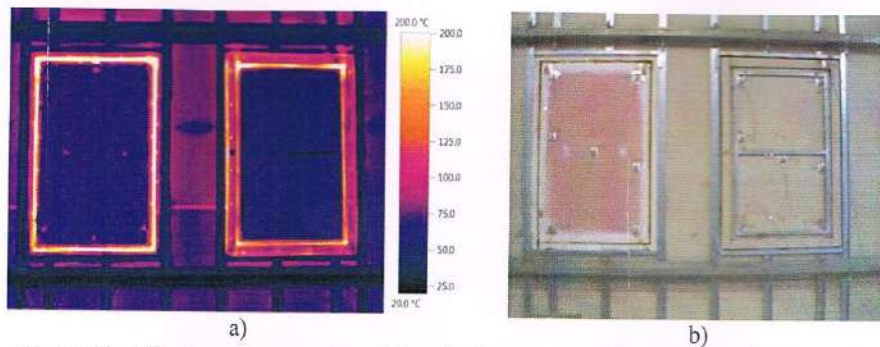
Figura 19. a) Campo de temperaturas; b) parte da amostra sujeito ao campo de temperaturas em a).
